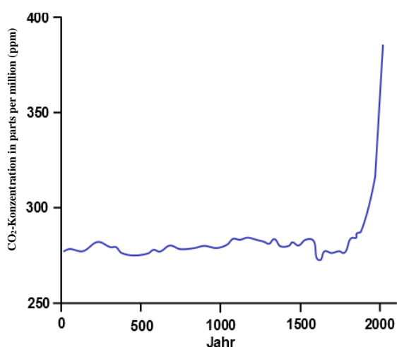
Abbildung 1: Zeitliche Änderung der \text{CO}_2 -Konzentration in der Erdatmosphäre von 0 bis 2012. Quelle: IPCC Synthesis Report 2013.
