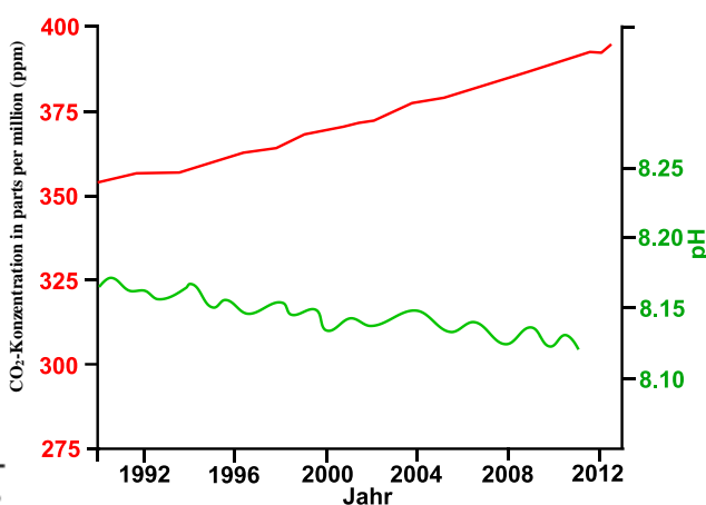
Abbildung 2: Zeitliche Änderung der \text{CO}_2 -Konzentration in der Erdatmosphäre von 1990 bis 2011 sowie die durchschnittliche pH-Änderung der Ozeane im selben Zeitraum. Quelle: IPCC Synthesis Report 2013.
